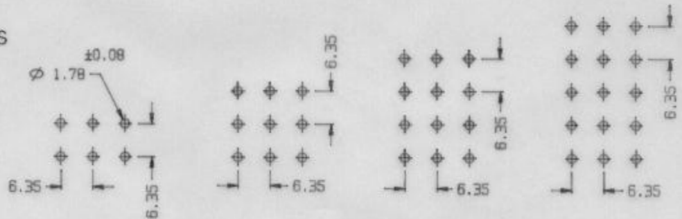
Padrao de furacao reconendada
